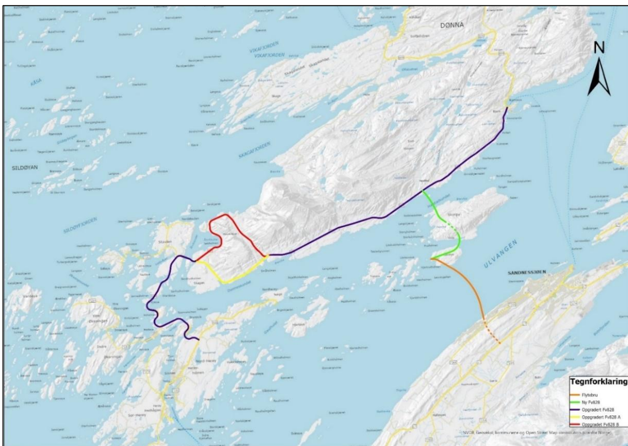
Kart 5: Alternativ 3 - Flytebru + oppgradering av eksisterende veg
