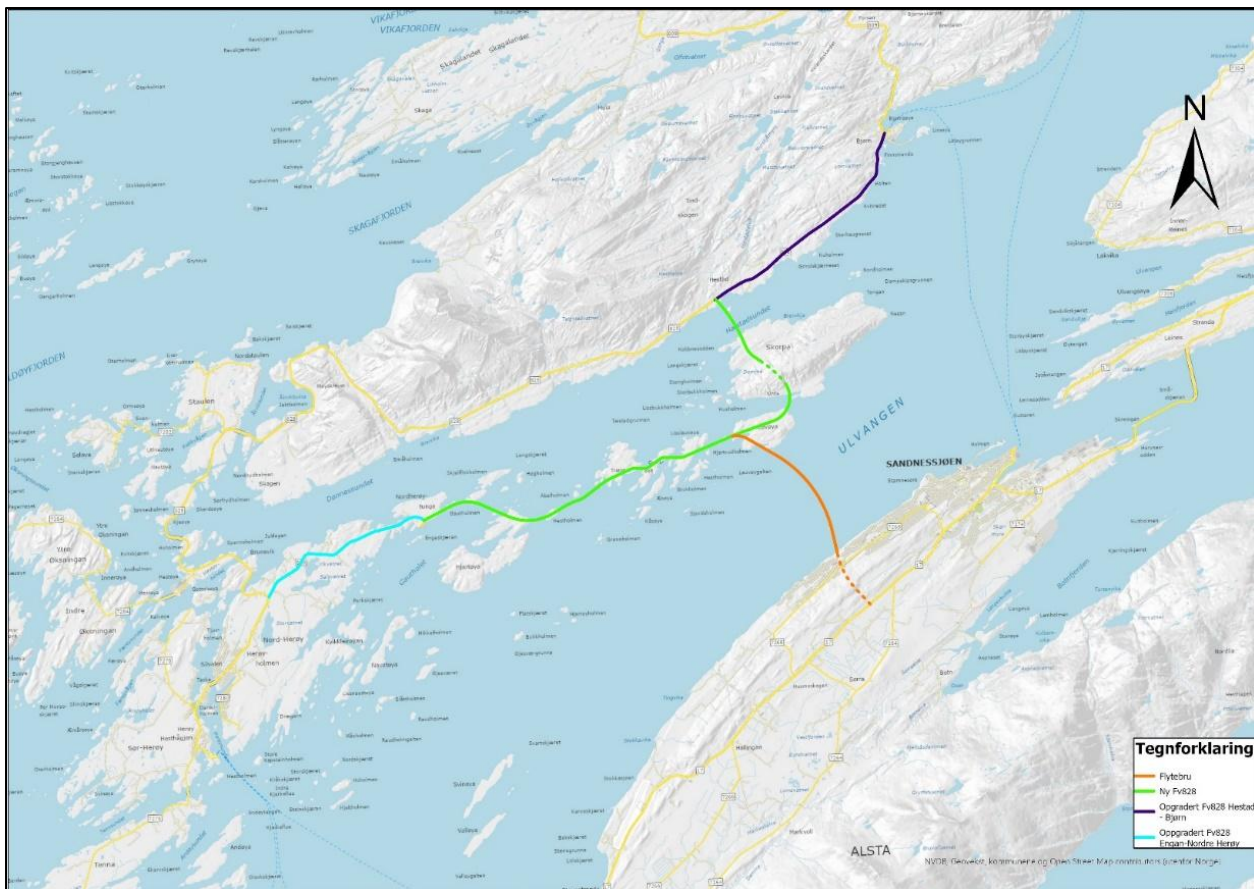
Kart 6: Alternativ 4 – Flytebru + ny veg mellom Engan og Hestad
