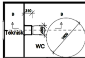
Prinsippskisse type 2
