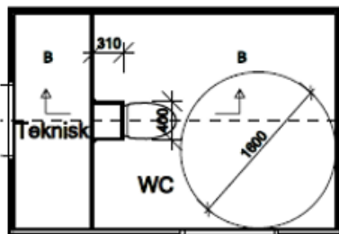
Prinsippskisse type 1
